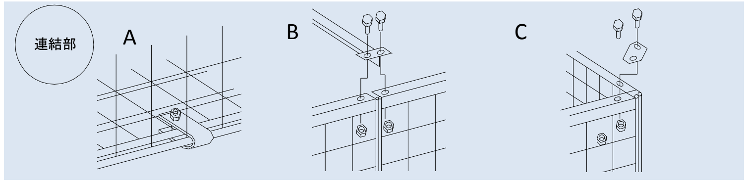
A: 平板クリップ取付部
